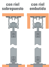
VISTA LATERAL PUERTA ABATIBLE
