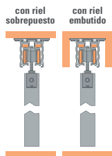
VISTA LATERAL PUERTA CORREDERA
