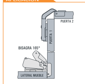
La puerta queda sobrepuesta ajustada al canto, A 165°.
