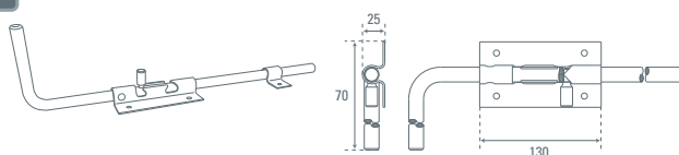
Picaporte para portón de acero zincado DUCASSE
