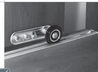
Sistema CORREDIZO AL SUELO con freno para puertas sobrepuestas de madera o marco de aluminio.
