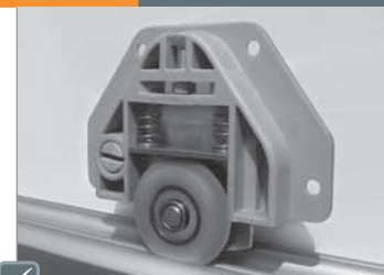
Sistema CORREDIZO AL SUELO con freno para puertas de closet. Con regulación de altura constante, gracias a sus dos resortes.
