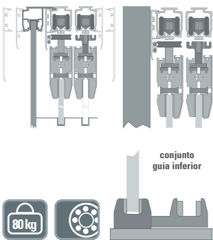
montaje con riel paño fijo superior e inferior
