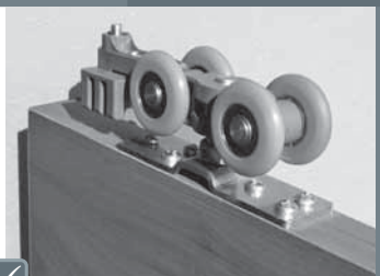
Sistema CORREDIZO COLGANTE con freno para puertas de madera.
