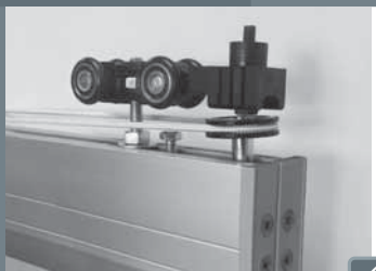
Sistema CORREDIZO COLGANTE para puertas de vidrio.
