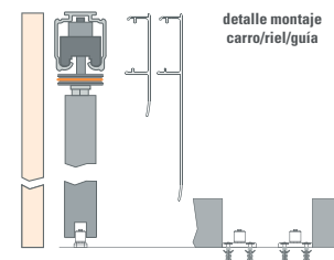
instalación a muro
