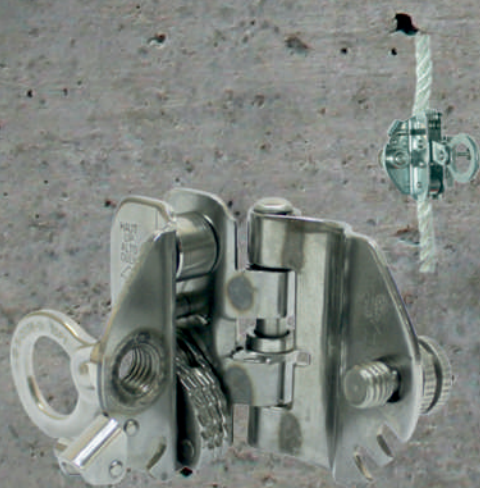
DESLIZADOR DESMONTABLE
